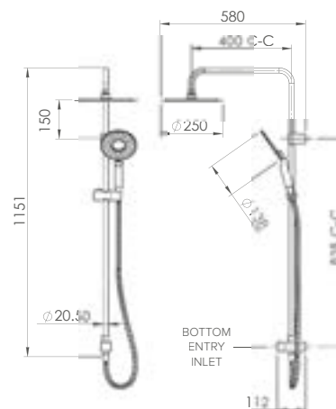
HRSCC BOTTOM ENTRY INLET
